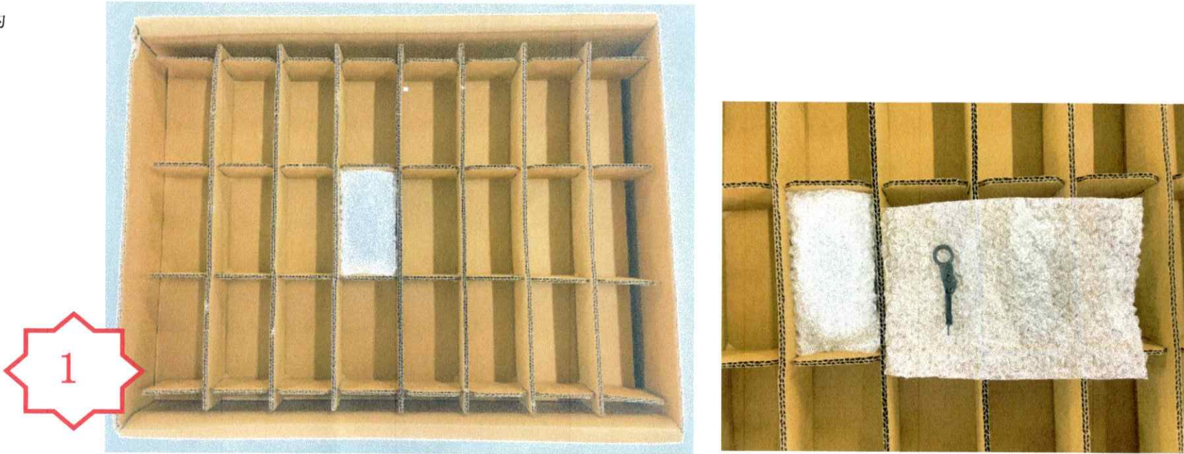
图一，每 10 个组件用一个小气泡袋装，每格 3 袋，每格 30pcs，每层 24 格，每层 720pcs，共 3 层，满箱 2160pcs
